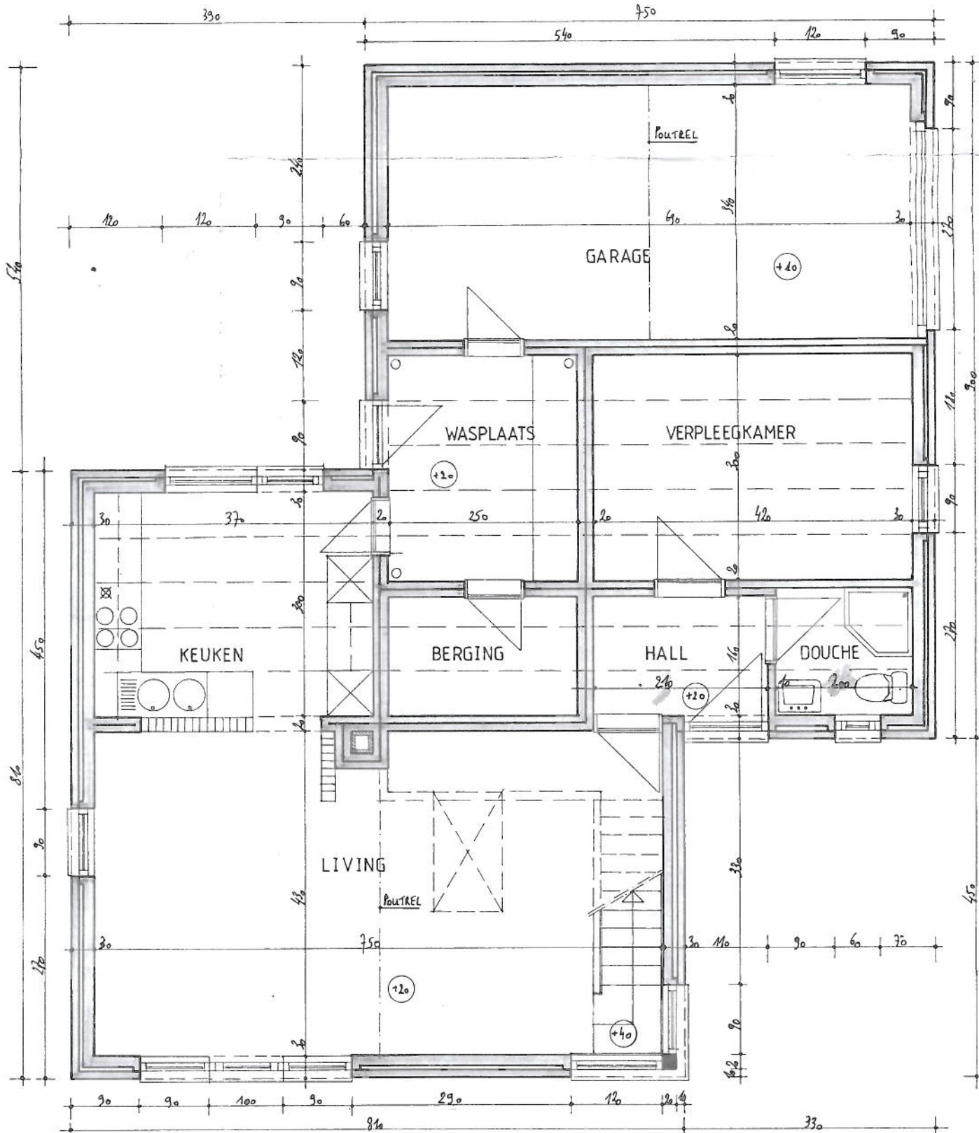
plan GELIJKVLOERS
